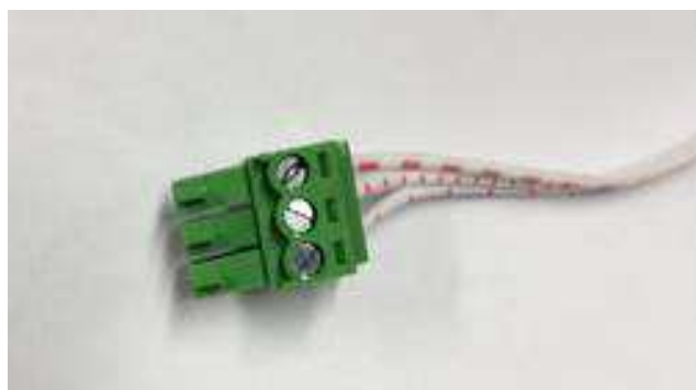
Рис. 5 Коннектор ИК-приемника
